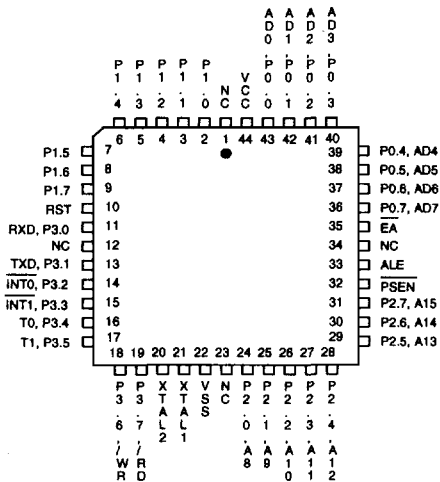
44-Pin PLCC (W78C31BP)
