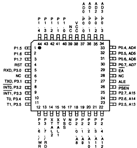
44-Pin QFP/TQFP (W78C31BF/W78C31BM)
