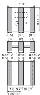
CSACV_X_Q 20.01-70.00MHz
