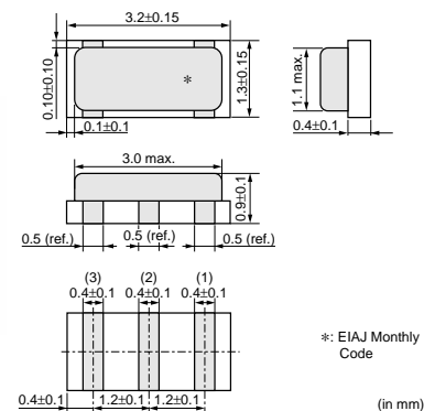
CSTCE_V13C 14.00-20.00MHz
